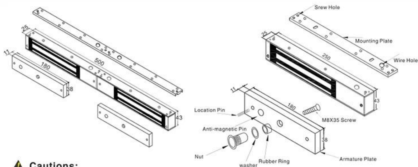
Diagram(unit:mm)
